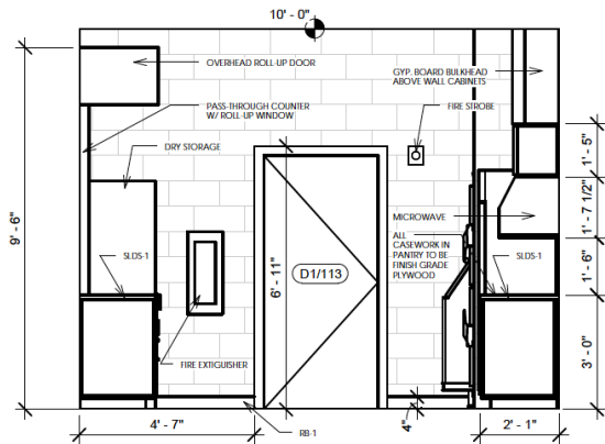
A4 PANTRY C 3/8" = 1'-0"
